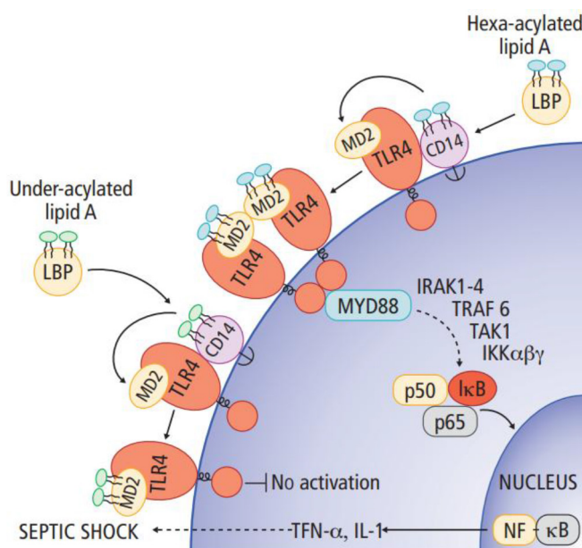
تصویر شماره ۲- بر همکنش اندوتوکسین با پروتئین متصل شونده به لیپوپلی ساکارید (LBP) و مولکول‌های سطح سلول MD2, CD14 و گیرنده شبه TLR4 (TLR4) (۵).
