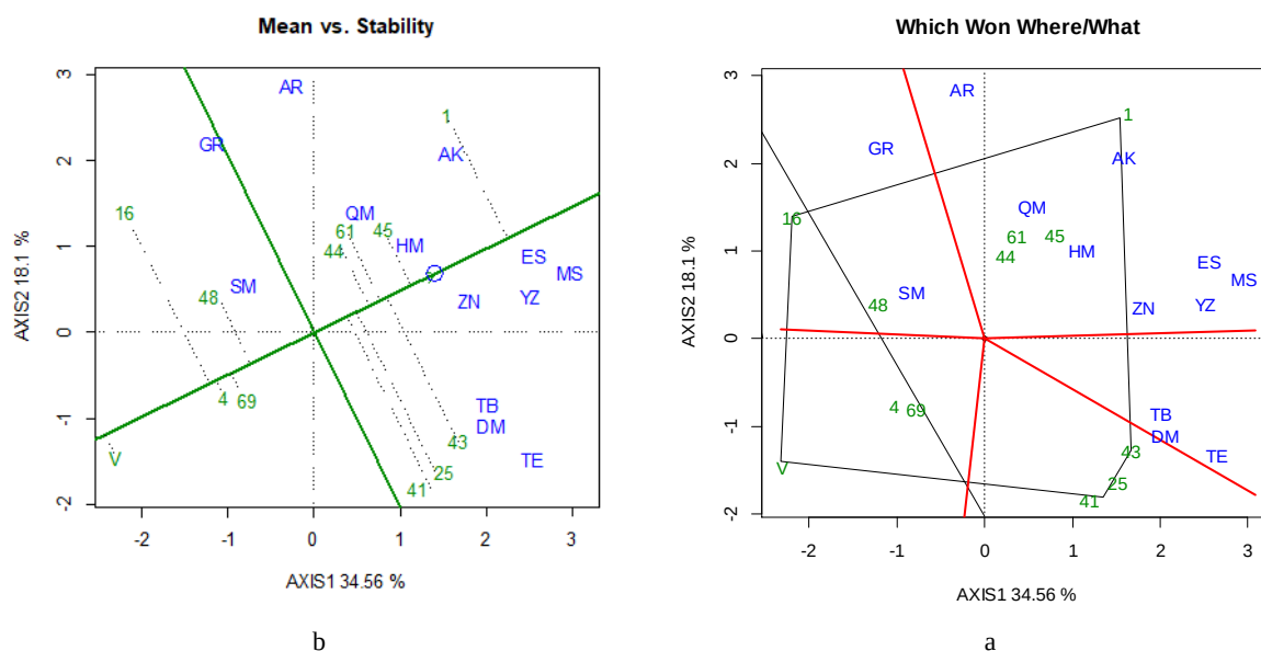
شکل ۲- a) نمودار بای پلات چندضلعی برای تعیین بهترین ژنوتیپ در هر محیط و b) نمودار بای پلات گزینش همزمان درصد اسانس و پایداری ژنوتیپ‌های Th. Lacnifolius براساس خط مختصات میانگین محیط (AEC) نام کامل مکان‌ها در جدول ۴ نشان داده شده است.
