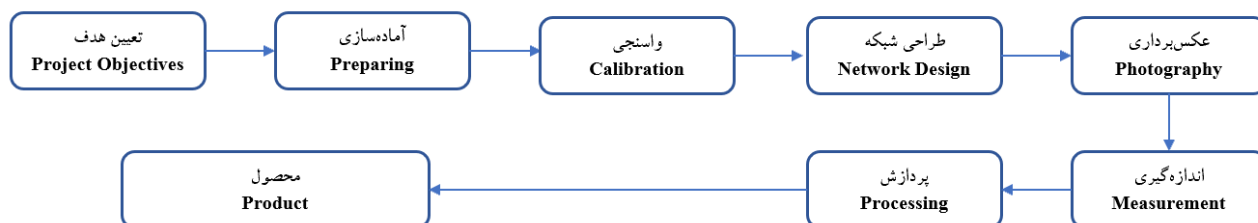
شکل ۲- فلوچارت مراحل کلی اجرای یک پروژه تصویرسنجی
