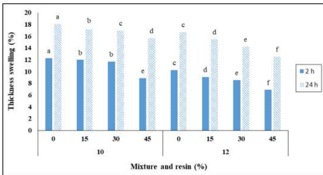
شکل ۵- اثر اختلاط و رزین بر واکنشیدگی ضخامت تخته‌ها بعد از ۲ و ۲۴ ساعت غوطه‌وری در آب Figure 5. The effect of mixture and resin on thickness swelling after 2 h and 24 h immersion in water
