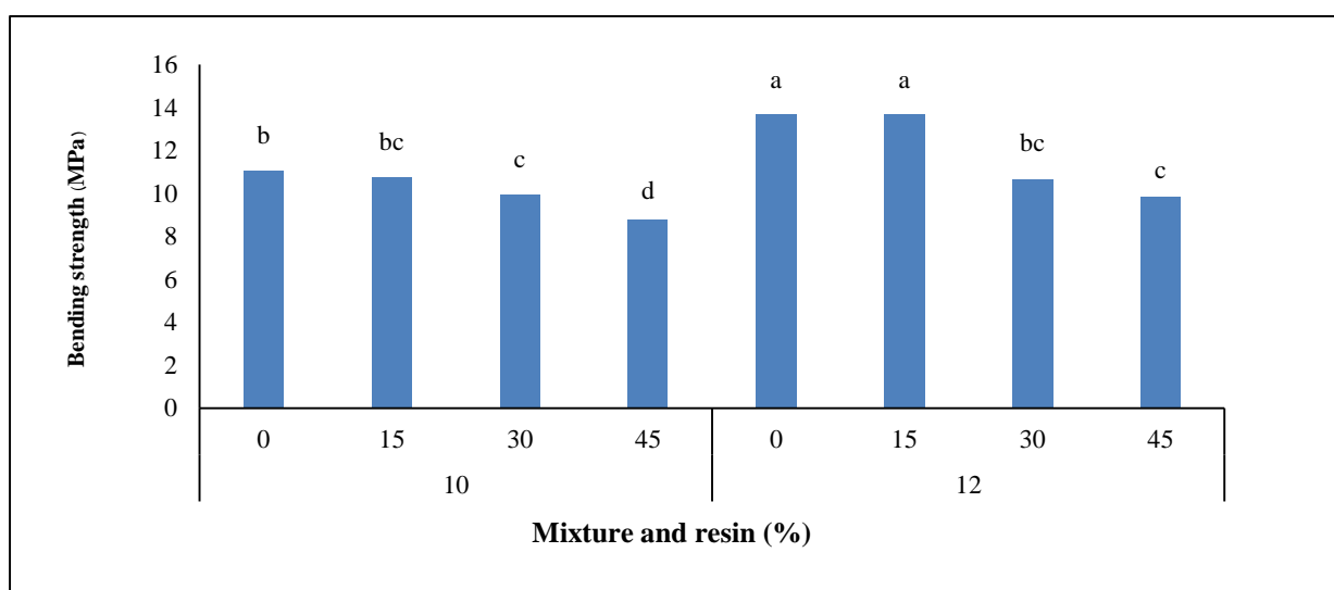
شکل ۱- اثر اختلاط و رزین بر مقاومت خمشی
