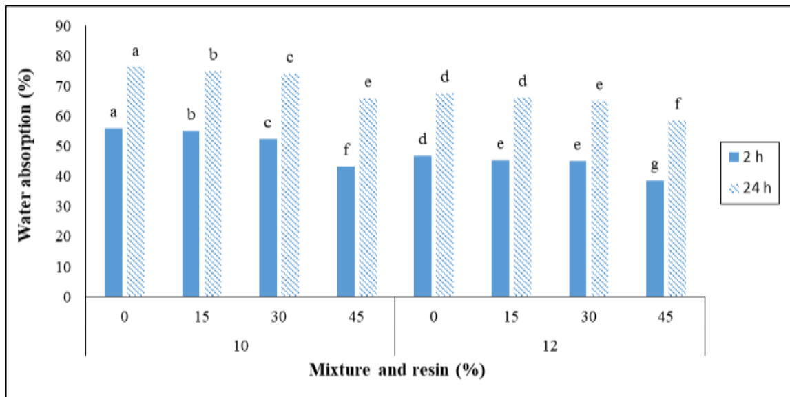
شکل ۴- اثر اختلاط و رزین بر جذب آب تخته‌ها بعد از ۲ و ۲۴ ساعت غوطه‌وری در آب
