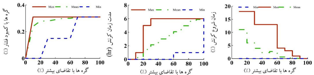
شکل ۱۹- اندازه کرنش، مدت زمان کرنش، زمان شروع کرنش سناریو افزایش قطر لوله (ساعات ۱۸ تا ۲۱) Fig. 19. Strain magnitude, strain duration and time of strain of increasing pipe diameter (period under stress: hours 18-21)
