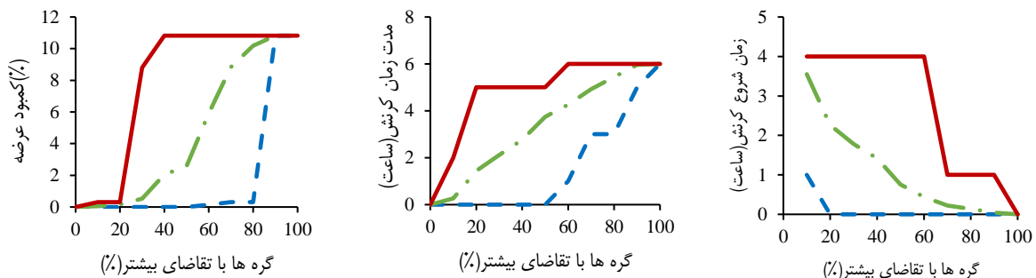
شکل ۱۵- نتایج شبیه‌سازی نیاز اضافی برای شبکه کنگاور در ساعات ۱۸-۲۱
