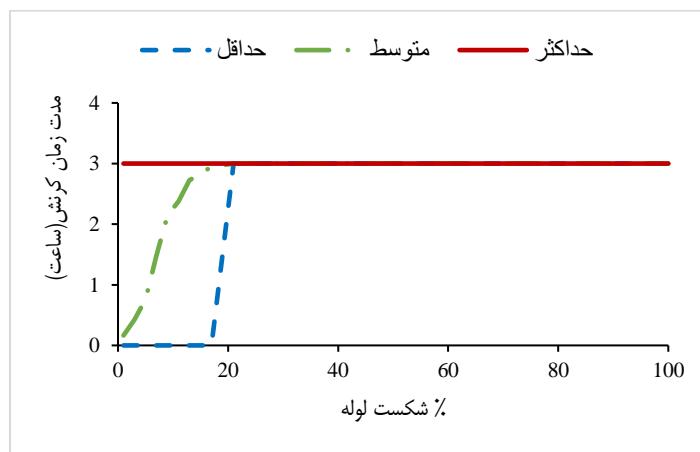
شکل ۷- نتایج مدت زمان کرنش برای شبکه آبرسانی Net3
