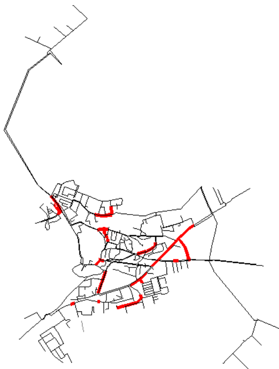
شکل ۱۸ - شبکه کنگاور - موقعیت لوله‌های با افزایش قطر
