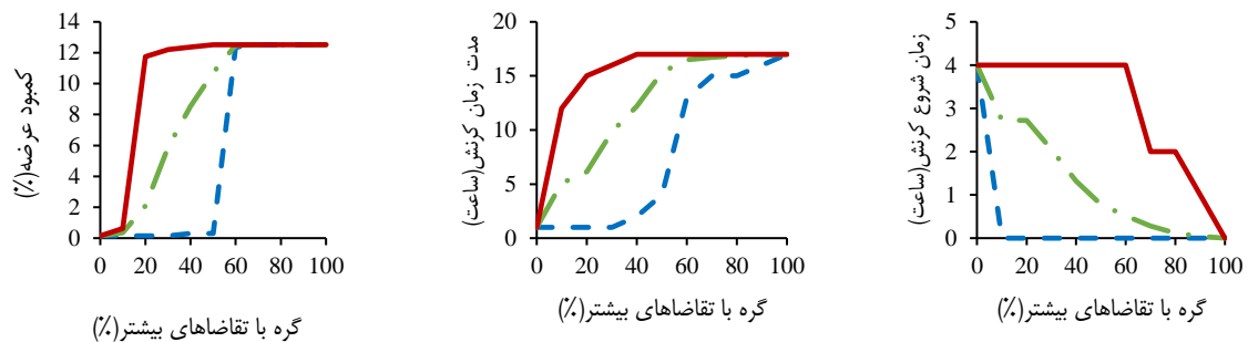
شکل ۱۶- نتایج شبیه‌سازی نیاز اضافی برای شبکه کنگاور (در ساعات ۹-۱۲)
