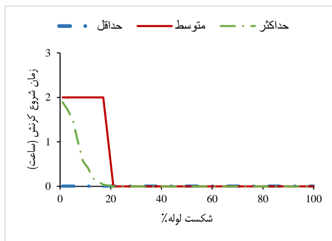
شکل ۸- زمان شروع کرنش برای Net3
