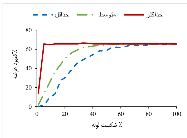
شکل ۹- نتایج اندازه کرنش برای شبکه کنگاور
