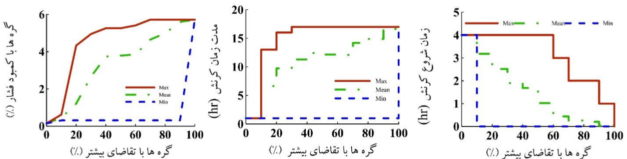
شکل ۲۰- اندازه کرنش، مدت زمان کرنش، زمان شروع کرنش سناریو افزایش قطر لوله (ساعات ۹ تا ۱۲) Fig. 20. Strain magnitude, strain duration and time of strain of increasing pipe diameter (period under stress: hours 9-12)
