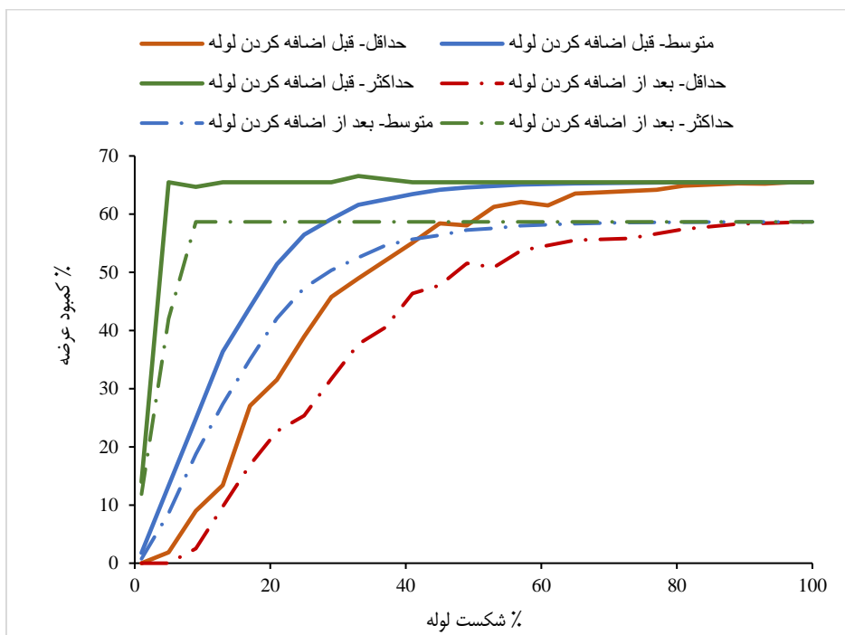
شکل ۱۲- مقایسه نتایج کمبود عرضه: قبل از اضافه کردن لوله و بعد از اضافه کردن لوله برای شبکه کنگاور
