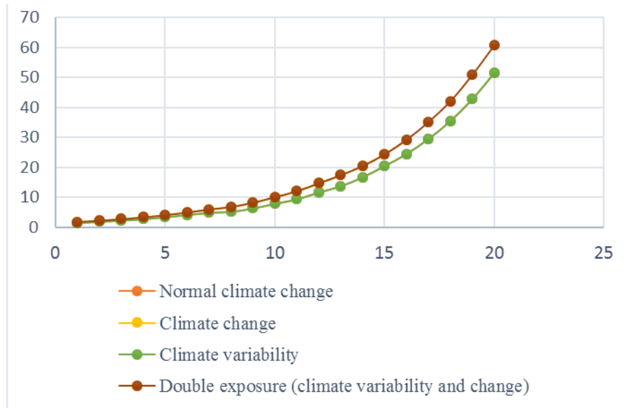
شکل ۴. قیمت هر تن محصول گندم ناشی از تغییرات اقلیمی Figure 4. Price per ton of wheat crop due to climate change منبع: یافته‌های پژوهش
