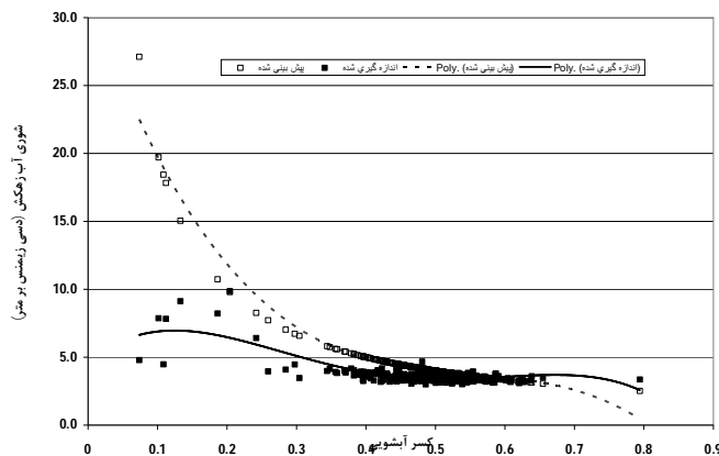
شکل 2- تاثیر کسر آبشویی بر حصول شرایط ماندگار
