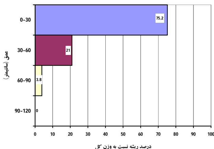
شکل 4- توزیع وزن ریشه در اعماق مختلف برای لایسیمتر شماره 13
