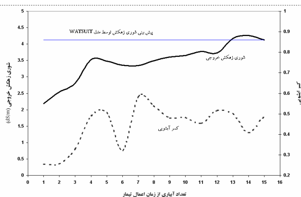
شکل 1- تغییرات شوری آب زهکش در مقابل تعداد دور آبیاری برای تیمار کسر آبشویی 50 درصد و شوری آب آبیاری 2 دسی زیمنس بر متر
