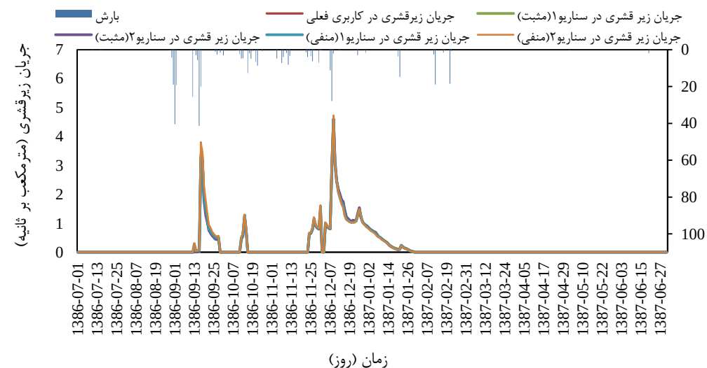
شکل ۱۱- نمودار جریان زیرقشری در کاربری فعلی و چهار سناریو در سال آبی ۱۳۸۶-۱۳۸۷
