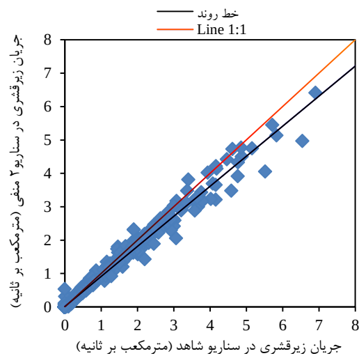
شکل ۱۶- نمودار مقایسه جریان زیرقشری در سناریو دو منفی و سناریو شاهد نسبت به خط ۱:۱
