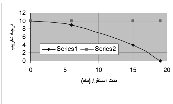
۱- Series 1 نمونه های دوام طبیعی و Series 2 نمونه های اشباع شده می باشد.
