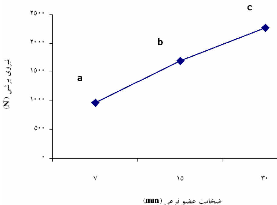
شکل ۱۱- تأثیر ضخامت عضو فرعی بر بار برشی اتصال در اتصالات ساخته شده با عضو اصلی با ضخامت ۳۰mm و عضو فرعی با ضخامت‌های ۷ و ۱۵ و ۳۰mm.
