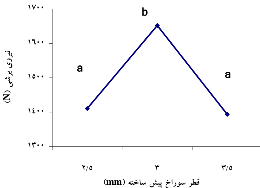
شکل ۶- تأثیر قطر سوراخ پیش ساخته بر مقدار بار برشی اتصال
