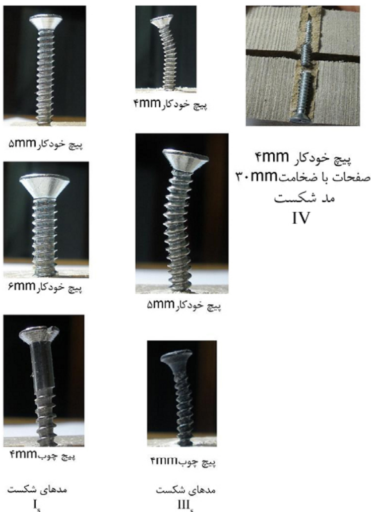
شکل ۳ - نمایی از تغییر شکل پیچ‌های مورد مطالعه زیر بار برشی (تمام پیچ‌هایی که با مد شکست I s و III s شکسته‌اند با ضخامت ۱۵mm آزمون شده بودند).
