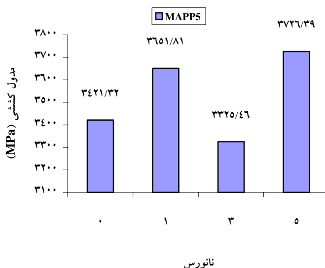
شکل ۱- تأثیر میزان نانورس بر مدول کششی
