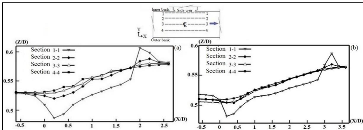
شکل ۶- تغییرات سطح آزاد شبیه‌سازی شده جریان در امتداد سرریز جانبی (a) L/D=2 و (b) L/D=3
