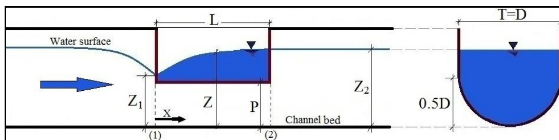
شکل ۳- طرح شماتیک کانال U شکل دارای سرریز جانبی مورد مطالعه اویماز (Uyumaz, 1997)
