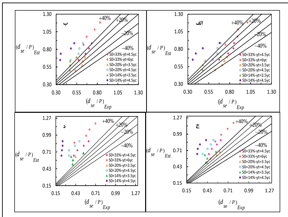
شکل ۱۴- مقایسه مقادیر اندازه‌گیری شده و برآورد شده حداکثر عمق نهایی آب‌شستگی، برای شیب و عمق‌های پایاب مختلف:
