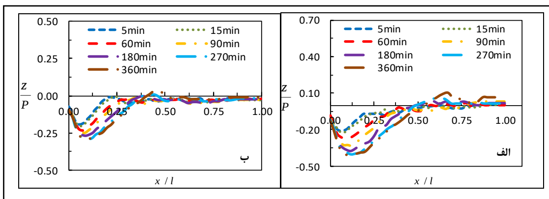
شکل ۷- نیمرخ لحظه‌ای تغییرات بستر در پایین دست سطح شیب دار برای شیب کارگذاری ۱۴ درصد، \eta = 10 و y_t = 4/5 y_c (ب) ، \eta = 15 و y_t = 3/5 y_c (الف) و عمق‌های پایاب مختلف: k_s = 10 \text{ mm} ، q = 28/4 \text{ l/s/m}
