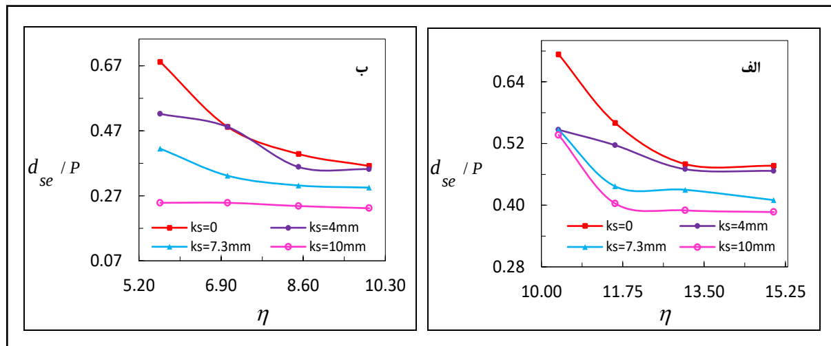
شکل ۱۳- مقایسه مقادیر حداکثر عمق نهایی آبشستگی برای شیب ۱۴ درصد، \eta و زبری های مختلف: الف) y_t = 3/5 y_c و ب) y_t = 4/5 y_c
