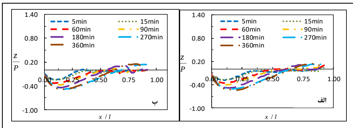
شکل ۶- نیمرخ لحظه‌ای تغییرات بستر در پایین دست سطح شیب دار برای شیب کارگذاری ۲۰ درصد، \eta = 9/5 و y_t = 4/5 y_c (ب) ، \eta = 15/2 و y_t = 3/5 y_c (الف) و عمق‌های پایاب مختلف: k_s = 7/3 \text{ mm} ، q = 34/1 \text{ l/s/m}
