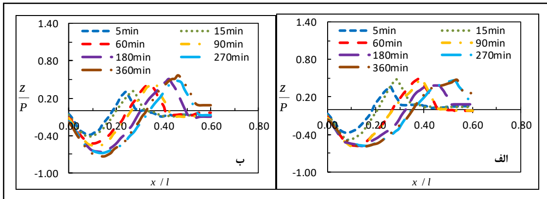
شکل ۵- نیمرخ لحظه‌ای تغییرات بستر در پایین دست سطح شیب دار برای شیب کارگذاری ۳۳ درصد، \eta = 2/6 و y_t = 6 y_c (ب) ، \eta = 8/8 و y_t = 4/5 y_c (الف) و عمق‌های پایاب مختلف: k_s = 4 \text{ mm} ، q = 39/8 \text{ l/s/m}
