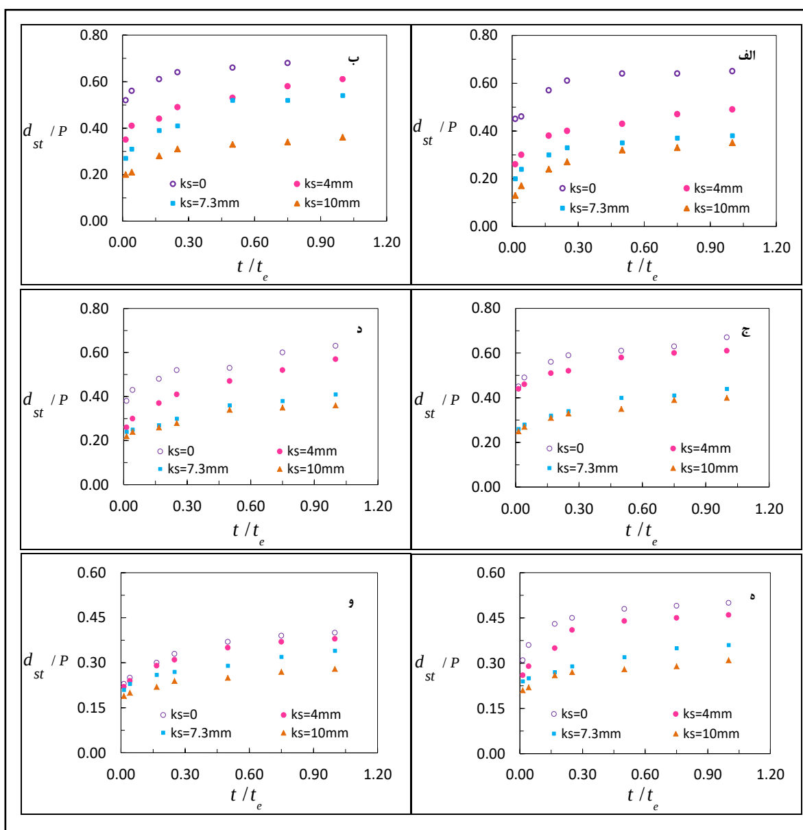
شکل ۱۰- توسعه زمانی حداکثر عمق لحظه‌ای آب‌شستگی برای دبی واحد عرض ۲۸/۴ لیتر بر ثانیه بر متر،
