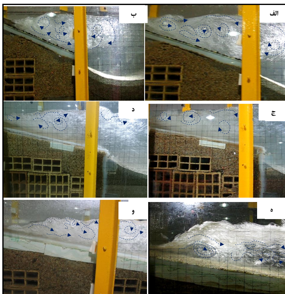
شکل ۸- نمایی از گردابه‌های تشکیل شده روی سازه کنترل تراز بستر سطح شیب‌دار برای شیب و عمق‌های پایاب مختلف:
