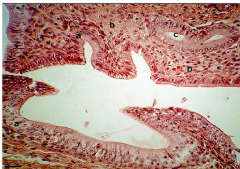
شکل ۱۲- دی ماه. محل اتصال رحم به واژن. b پارین، c لوله ذخیره کننده اسپرم. رنگ آمیزی هماتوکسیلین - ائوزین 240 \times 12 \mu\text{m} . Scale=
