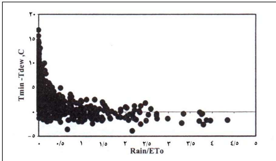
شکل شماره ۱- نمودار T_{\min} - T_{\text{dew}} در مقابل \text{Rain}/\text{ET}_0 ، بررسی سالانه، مشهد
