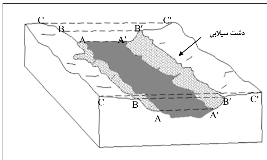
شکل شماره ۱ - سطوح مرجع نهشته رسوبی (C-C') سطح مرجع کانال فعال (B-B') مقطع پر (A-A') شکل شماره ۱ - سطوح مرجعی که برای توسعه روابط ژئومتری-کانال در بریتانیا مورد استفاده است [۱۳]
