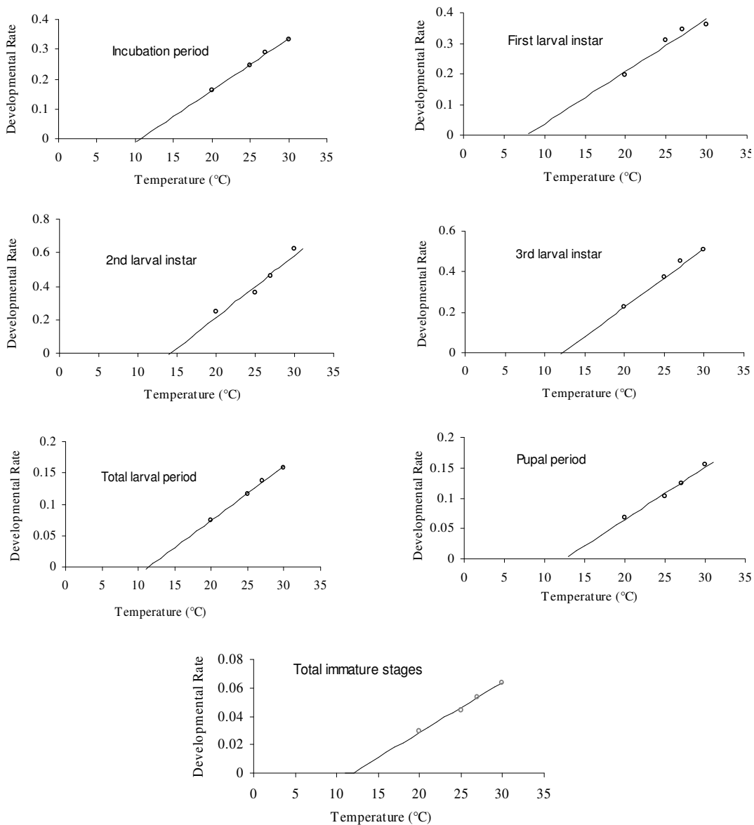
شکل ۱- برازش مدل خطی معمولی روی مقادیر مشاهده شده نرخ رشد و نمو مراحل زیستی نابالغ بالتوری سبز معمولی Chrysoperla carnea در دماهای مورد بررسی. نقاط توخالی، نرخ رشد و نمو مشاهده شده و خط، نشان دهنده مقادیر پیش بینی شده به وسیله مدل است.
