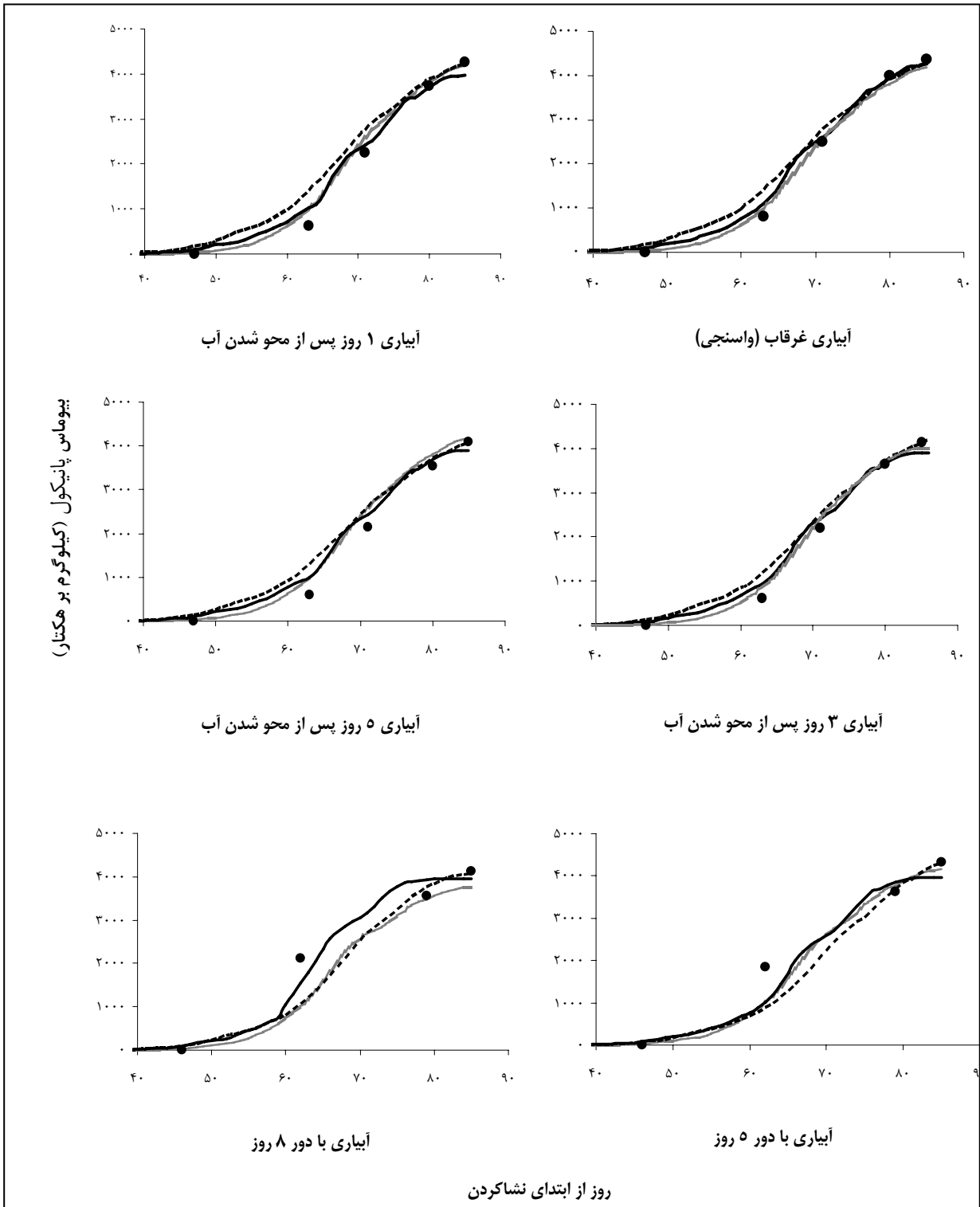
شکل ۲- مقایسه مقادیر شبیه‌سازی مدل‌های WOFOST (—)، SWAP (---) و ORYZA2000 (· · ·) و اندازه‌گیری بیوماس پانیکول در دوره‌ی رویش در مدیریت‌های آبیاری (●)
